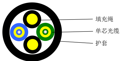
双芯圆形基站光缆 I 型
